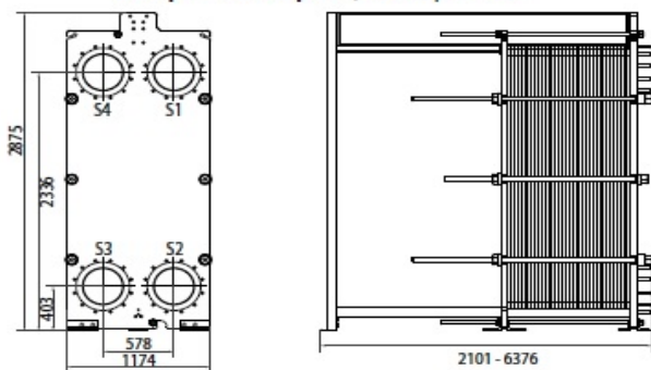
Габаритный чертеж, Размеры в мм
